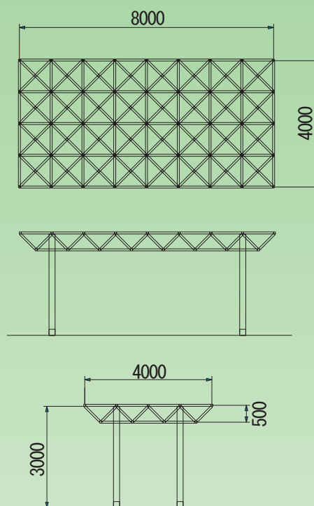
■木造トラスパーゴラ
